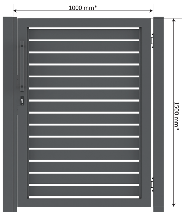
Furtka standartowa
