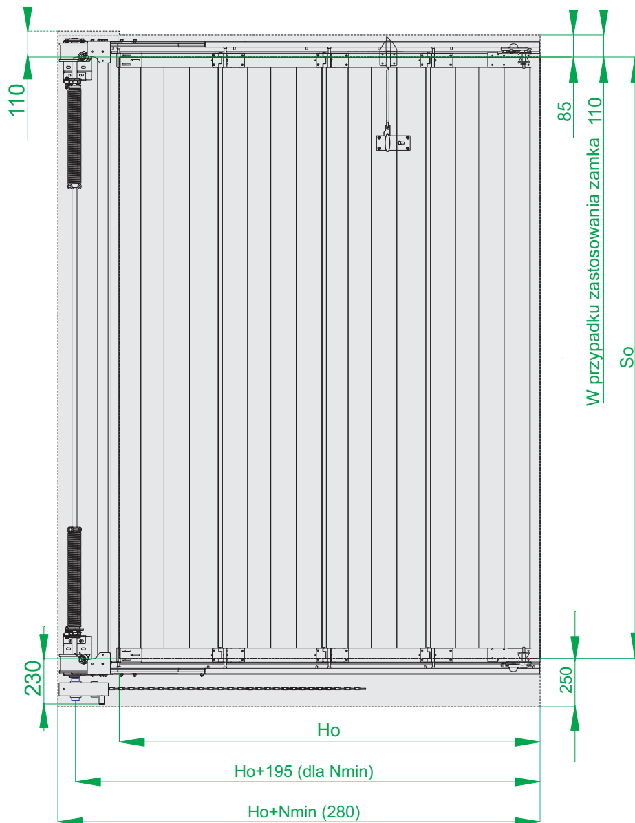
Brama z przekładnią łańcuchową
